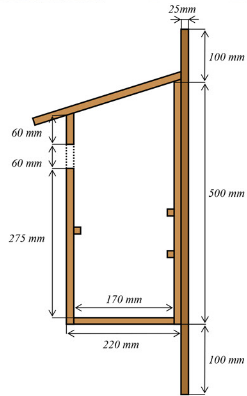
Inkilo kukučiams brėžinys
